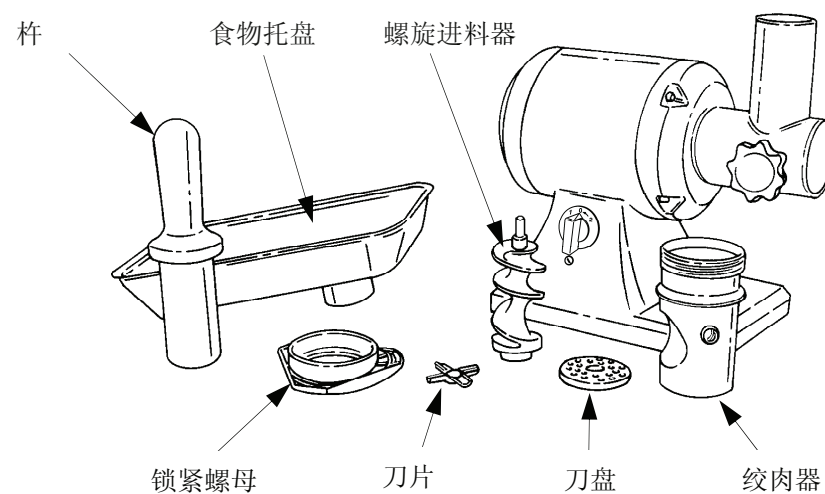
图10 - 清洗分解图
